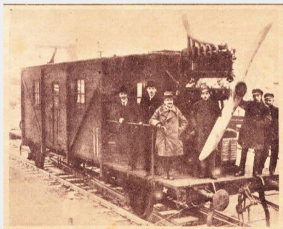
EEN NIEUWE UITVINDING. Dr. Ing. Otto Steinitz heeft een propeller-locomotief uitgevonden: twee vliegmotoren met 260 p.k. kunnen een snelheid van 130 K.M. per uur geven.
